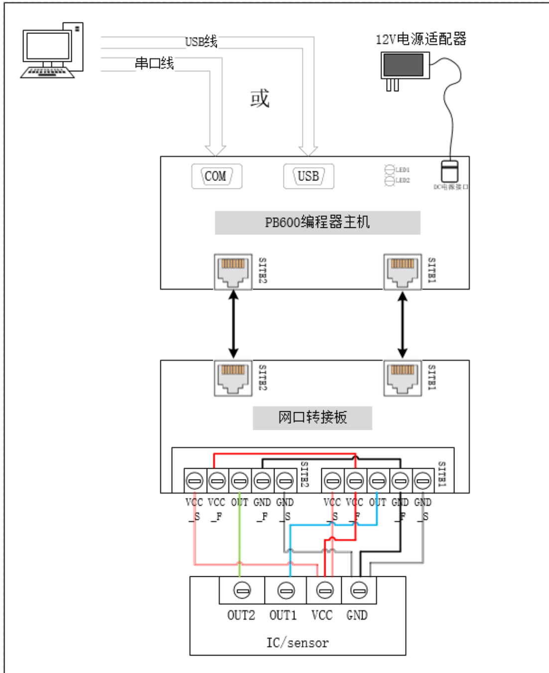
图3.2 PB600 编程器与1颗单电源供电的MT652xGT 芯片接线示意图
