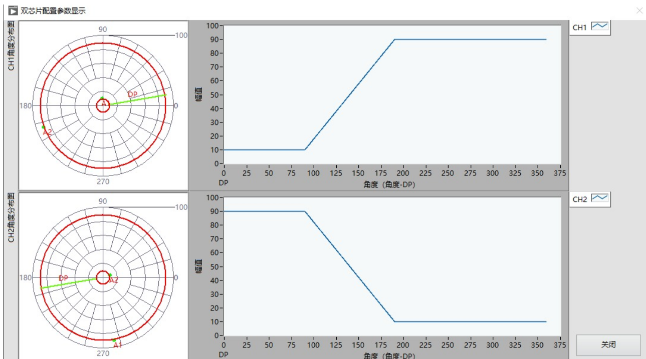
图 4.2.12 理论编程曲线图
