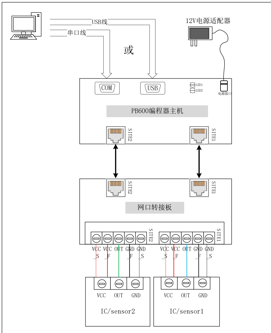
图3.1 PB600 编程器与2颗MT652xCT（或1颗MT652xGT）芯片接线示意图
